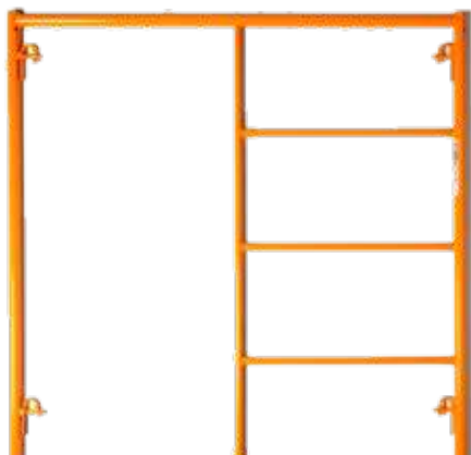
Marco de andamio de 2.00 x 1.00 mts
