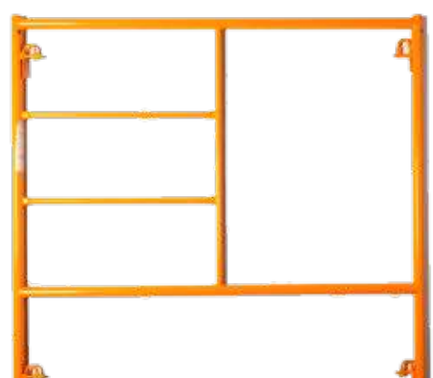
Marco de andamio de 2.00 x 1.55 mts
