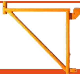
Escuadras para andamio de 60cms y 80cms.
